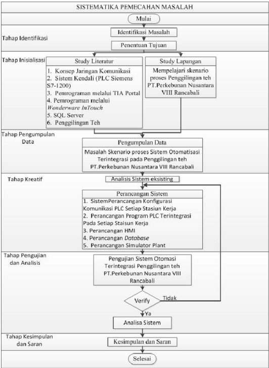
Gambar III. 1 Sistematika Pemecahan Masalah
