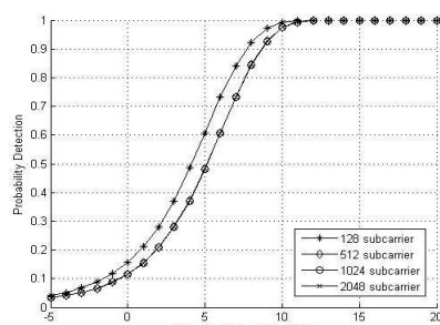
Gambar 4. Perbandingan P_d terhadap SNR
