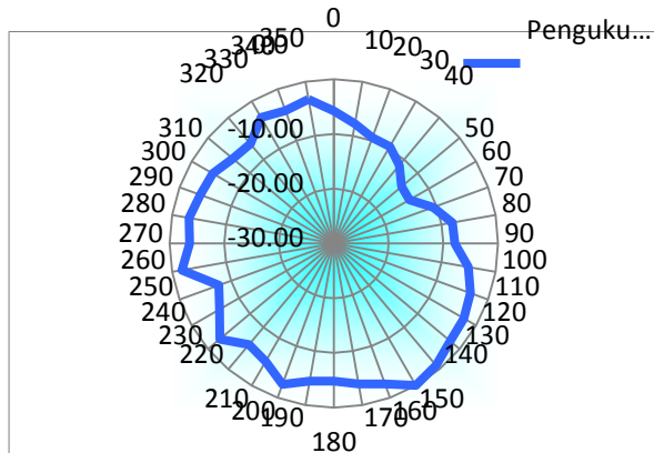
Gambar 14. Hasil Pengukuran Polaradiasi Azimuth
