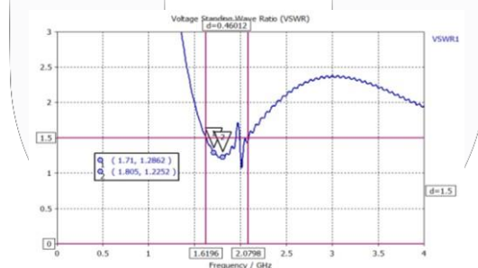
Gambar 3. Hasil Simulasi Antena VSWR
