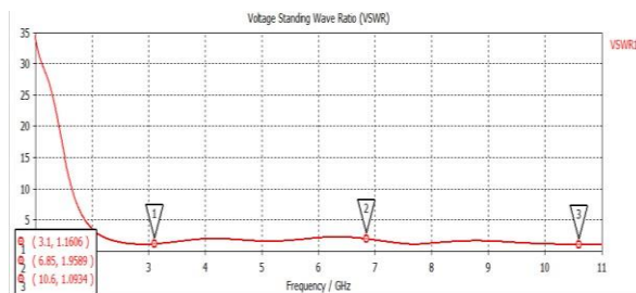
Gambar 6 (a) Grafik VSWR Pada Frekuensi ( 3.1 – 10.6) GHz di Free Space, (b) VSWR Antena pada Frekuensi (3.1-10.6) GHz saat Free Space
