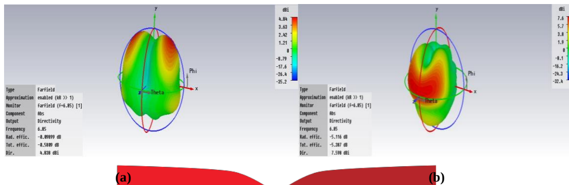
Gambar 9 (a) Gain Antena pada Frekuensi 6.85 GHz saat Free Space, (b) Gain Antena Pada Frekuensi 6.85 GHz saat Berada Dekat Phantom Sejauh 2mm
