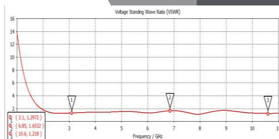
Gambar 7 (a) Grafik VSWR Pada Frekuensi ( 3.1 – 10.6) GHz, (b) VSWR Antena pada Frekuensi (3.1-10.6) GHz saat Berada Pada Phantom/Tubuh Manusia Sejah 2 mm
