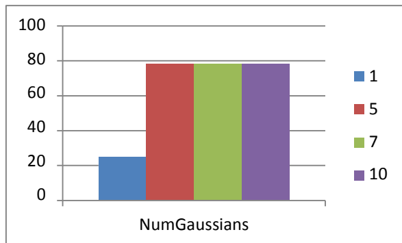
Gambar 4-3 Grafik NumGaussians
