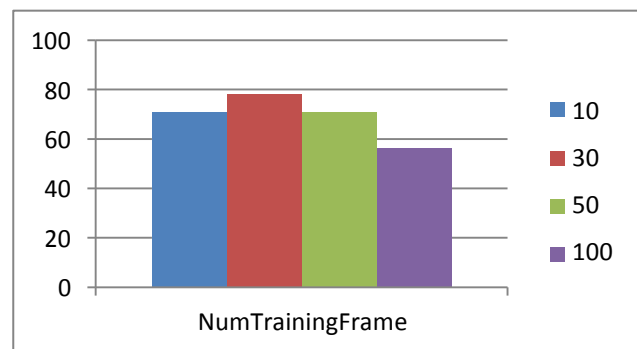
Gambar 4-2 Grafik NumTrainingFrame
