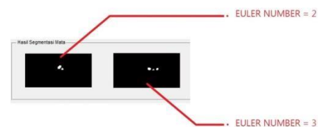
Gambar 3.5 Pengaplikasian EulerNumber
