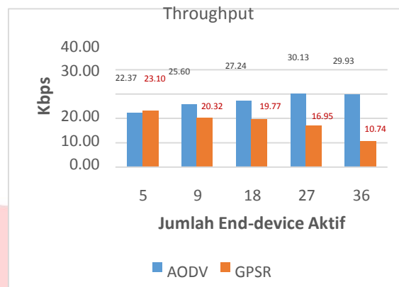
Gambar 4.2: Grafik nilai throughput berdasarkan kepadatan node pada skenario 1
