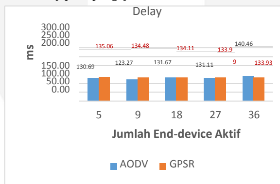
Gambar 4.1: Grafik rata-rata end-to-end delay berdasarkan kepadatan node pada skenario 1
