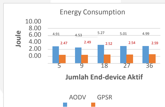
Gambar 4.3: Grafik nilai konsumsi energi berdasarkan kepadatan node pada skenario 1
