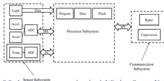
Gambar 2.2: Arsitektur umum pada sebuah Wireless Sensor Network [10]
