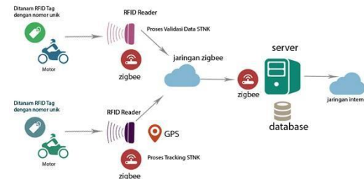
Gambar 3. 1 Desain Sistem
