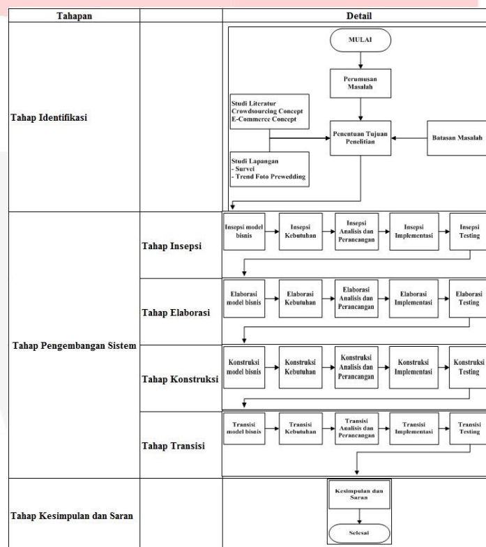
Gambar 2.3 Sistematika Penelitian
