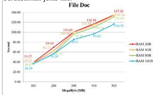
Gambar 4.5 Grafik Hasil Pengujian File Doc
