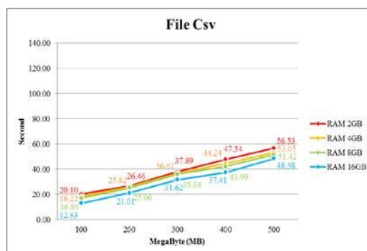
Gambar 4.7 Grafik Hasil Pengujian File Csv
