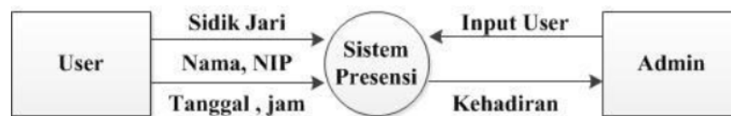
Gambar 3.3 DFD Sistem
