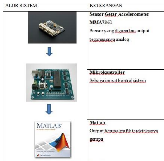
Gambar 3.1 Diagram Blok Sistem
