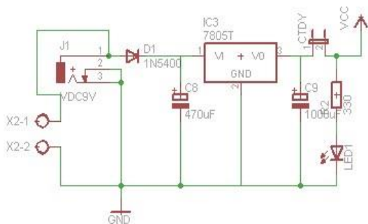
Gambar 3.5 Rangkaian Catu Daya
