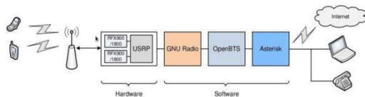
Gambar 2.1 Arsitektur Sederhana OpenBTS
