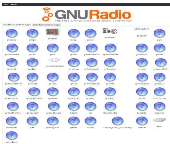
Gambar 2.3 Tampilan PyBOMBS
