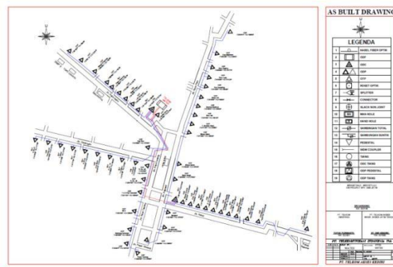
Gambar 3.2 Contoh hasil tagging
