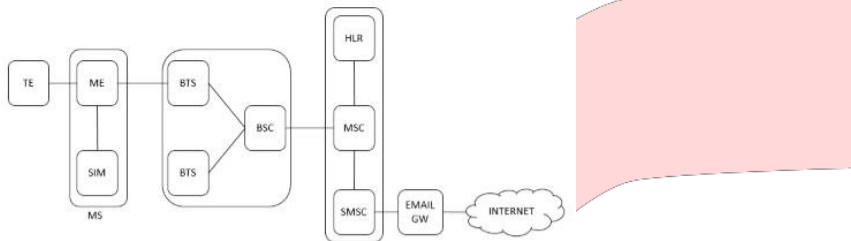
Gambar 2.1 Arsitektur SMS yang terintegrasi dengan jaringan GSM [1]
