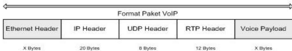
Gambar 1 Format Paket VoIP [8]
