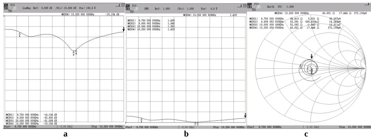
Gambar 10 Hasil Pengukuran a) Return Loss, b) VSWR, c) Impedansi
