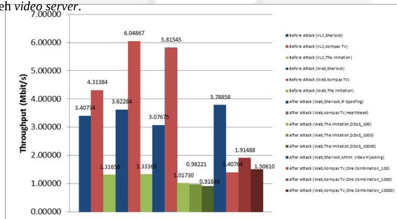
Gambar 4 – Nilai throughput setelah diserang
