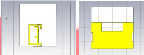
Gambar. 3.2 Antena tampak depan (kiri) dan tampak belakang (kanan)
