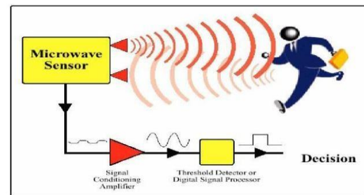
Gambar 3.2 Prinsip Kerja Sensor HB100
