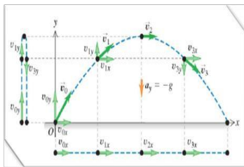
Gambar 2.1. Grafik Gerak Parabola
