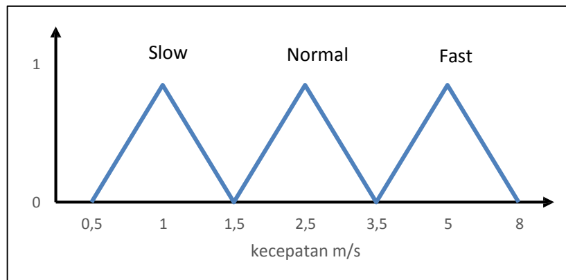
Gambar 7 Fungsi keanggotaan keluaran kecepatan
