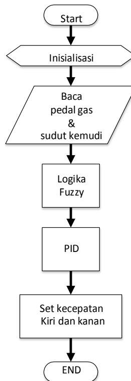
Gambar 3 Flowchart sistem kerja dan perancangan hardware
