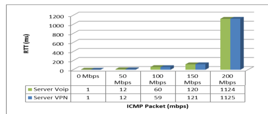
Fig. 2 Without VPN Soultion
