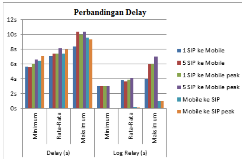
Gambar 3. Grafik Delay Pengiriman SMS
