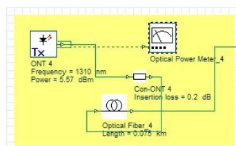
Gambar 6. Transmitter pada Link upstream pada Optisystem
