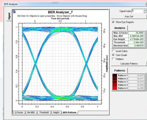
Gambar 4. BER Analyzer Optisystem pada link downstream
