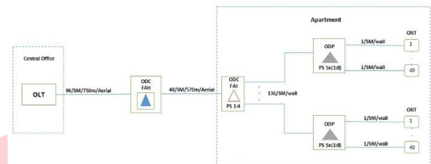
Gambar 2. Konfigurasi Umum Peletakan Perangkat FTTH (OLT-ONT)
