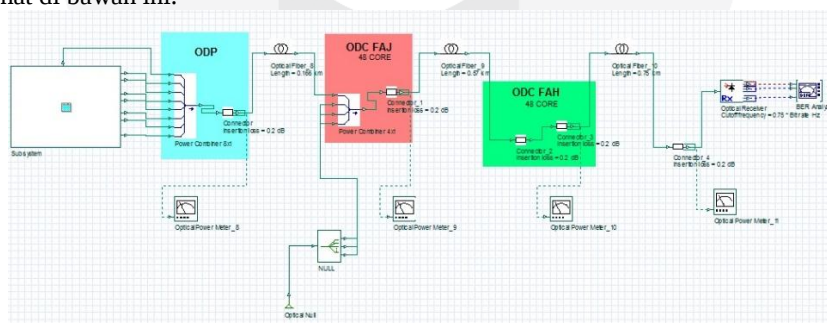
Gambar 5. Link upstream pada Optisystem
