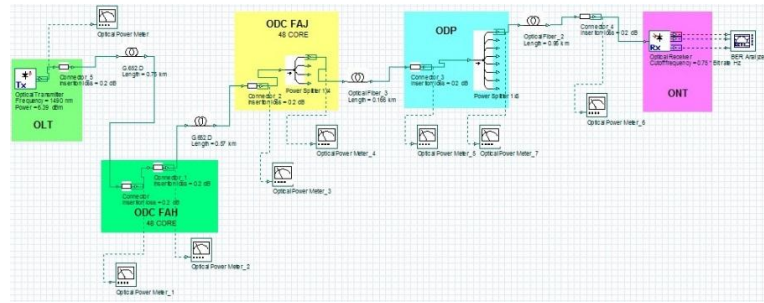
Gambar 3. Link downstream pada Optisystem
