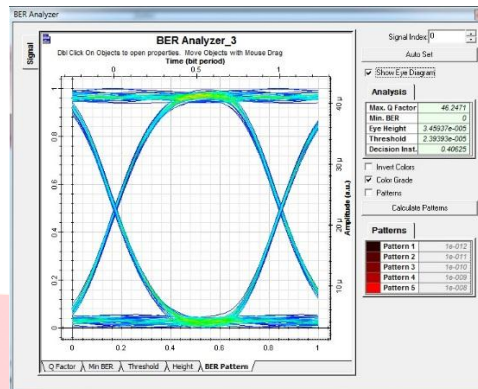
Gambar 7. BER Analyzer Optisystem pada link upstream
