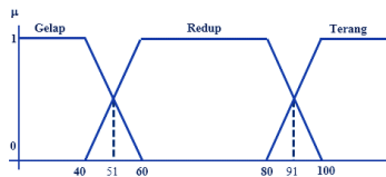
Gambar 7 Grafik Intensitas Cahaya
