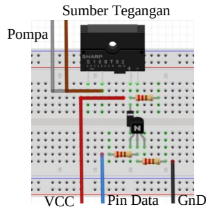
Gambar 92 Rangkaian Relay dan Pompa
