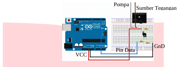
Gambar 10 Rangkaian Pompa dan Relay ke Arduino Uno
