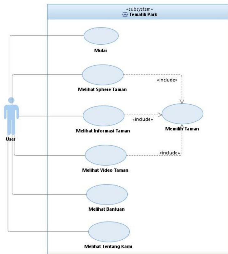
Gambar 3-2 Usecase Diagram Aplikasi Tematik Park
