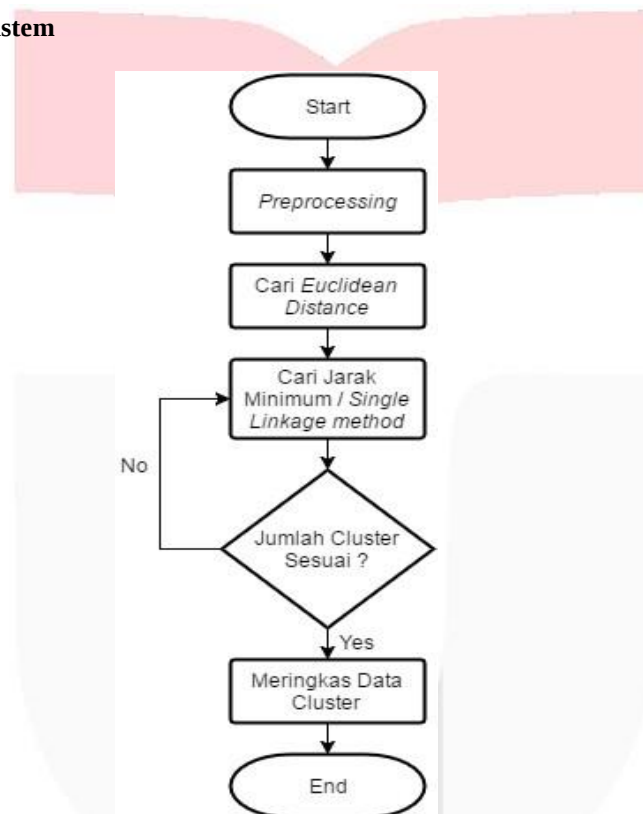
Gambar 2.1 Flowchart Umum Sistem
