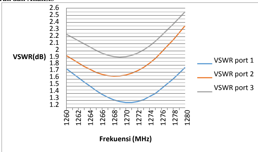
Gambar 4.1 Grafik VSWR
