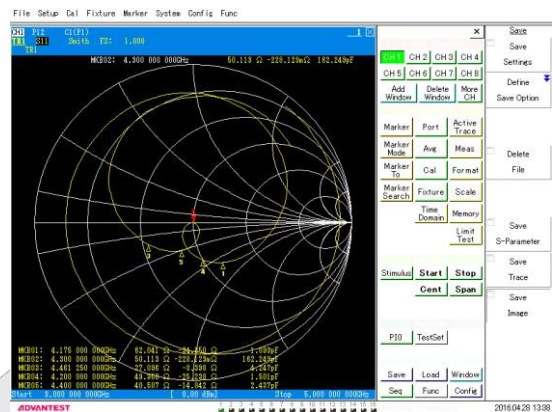
(b) Hasil Pengukuran Impedansi realisasi
