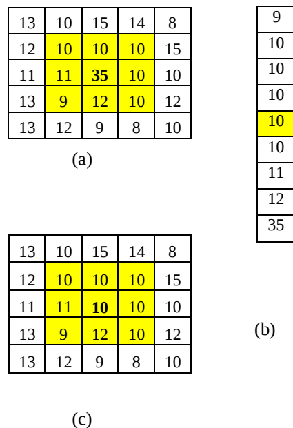
Gambar 1 (a) Matriks citra dengan window 3x3 , (b) Nilai intensitas citra setelah diurutkan, (c) Matriks citra hasil median filter.
