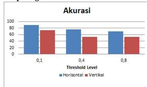
Gambar 7 Grafik Tingkat Akurasi pada Skenario 3
