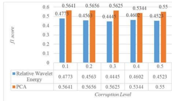
Gambar 10: Grafik performansi terbaik terhadap corruption level untuk kelas valence
