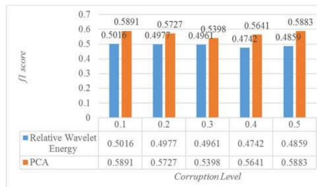
Gambar 12: Grafik performansi terbaik terhadap corruption level untuk kelas arousal
