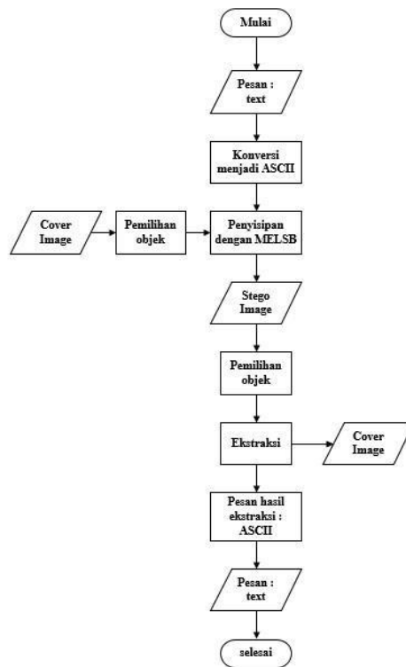
Gambar 1 Diagram Alir Perancangan Sistem Steganografi
