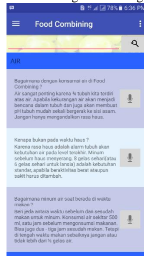
Gambar 8 Tampilan FAQ
