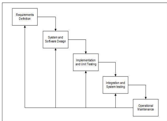
Gambar 1 Metode Pengerjaan
