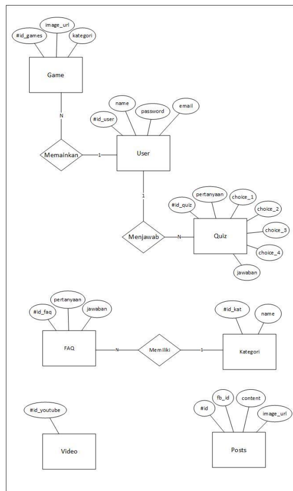
Gambar 3 ERD
