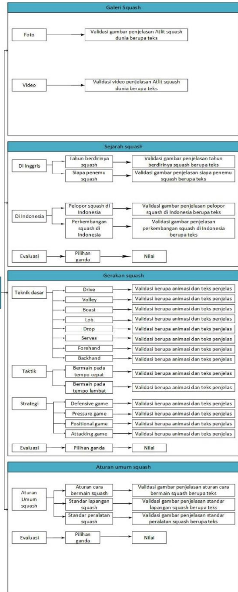
Gambar 9 Struktur instruksional
