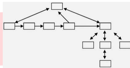
Gambar 4 Navigasi Komposit
