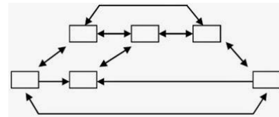
Gambar 3 Navigasi Nonlinear
