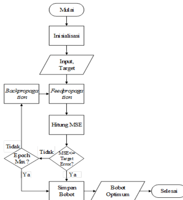
Gambar 3.9 Diagram Alir Pelatihan Jaringan Syaraf Tiruan-Backpropagasi
