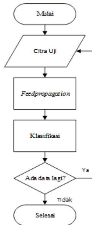
Gambar 3.10 Diagram Alir Pengujian Jaringan Syaraf Tiruan- Backpropagation
