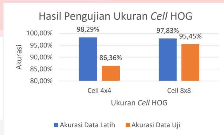
Gambar 2 : Hasil validasi ukuran cell HOG
