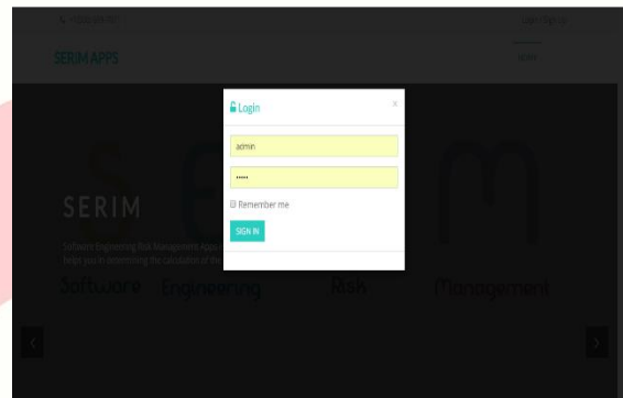
Gambar 4-1 Login Pengguna
