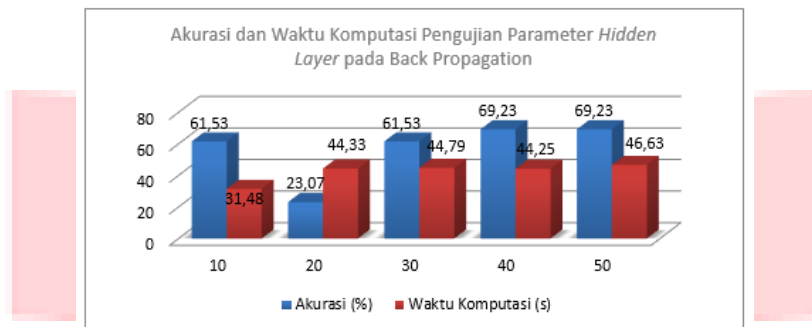
Gambar 12. Hasil Pengujian Parameter Hidden Layer pada JST-BP
