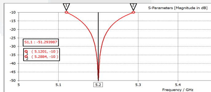
Gambar3.2 Antena Array 4 elemen setelah optimasi
