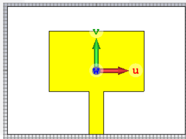
Gambar 1.4 Antena 1 elemen setelah optimasi
