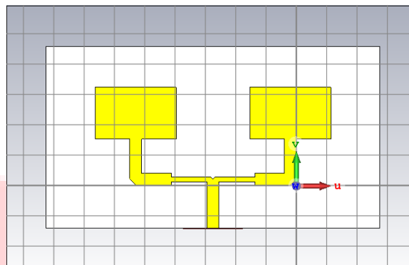
Gambar 1.5 Antena 2 elemen setelah optimasi
