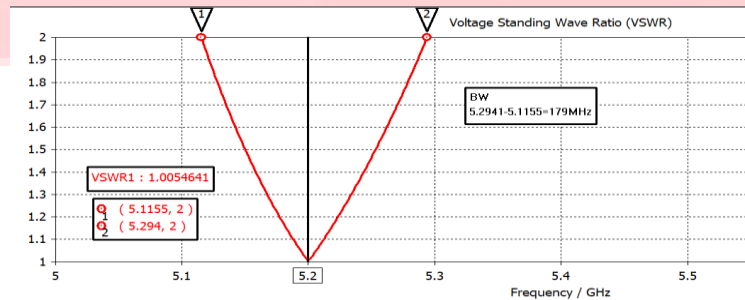
Gambar3.4 Bandwidth Antena 4 elemen setelah optimasi
