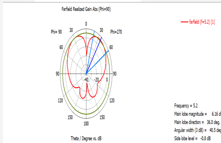
Gambar3.5 Pola Radiasi Antena 4 Elem Elevasi
