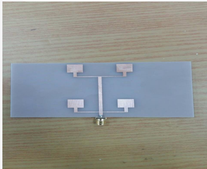
Gambar3.7 Realisasi Antena Planatr Array 2x2
