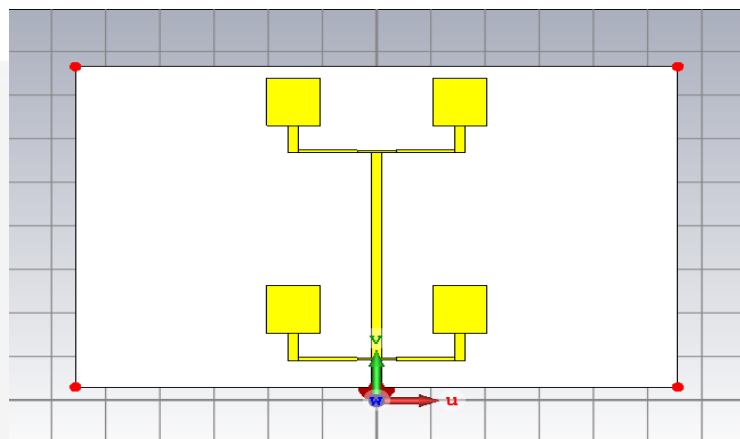
Gambar3.1 Antena Array 4 elemen setelah optimasi
