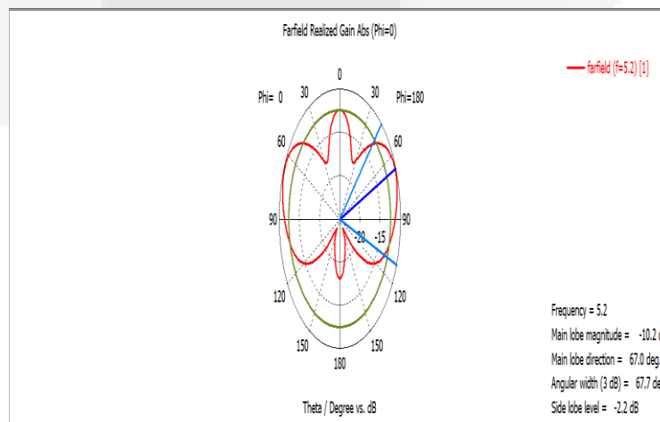
Gambar3.6 Pola Radiasi Antena 4 Elemen Azimuth
