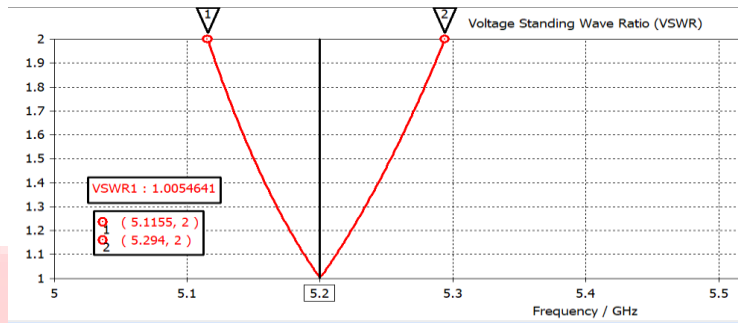
Gambar3.3 vswr Antena Array 4 elemen setelah optimasi
