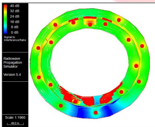
Gambar 3. 7 Simulasi SIR Skenario 2
