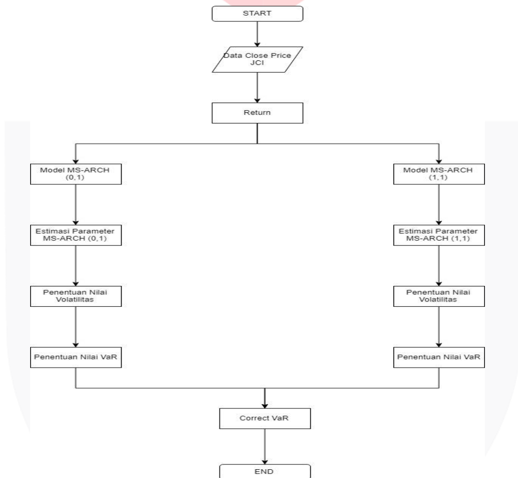
Gambar 1 Alur Perancangan Sistem prediksi Value-at-Risk menggunakan MS-ARCH
