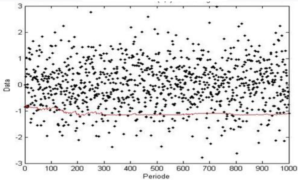
Gambar 3 Grafik Return dan VaR-MS-ARCH(1,1) Pada Tingkat Signifikansi 10%
