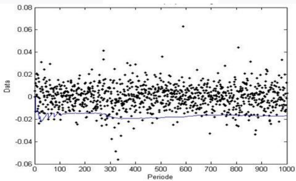
Gambar 1 Grafik Return dan VaR-MS-ARCH(0,1) Pada Tingkat Signifikansi 5%
