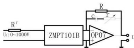
Gambar 2-1. Rangkaian Sensor ZMPT101B
