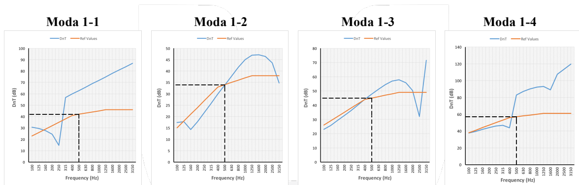
Gambar 6 Plot kurva D_{nT} dan kurva referensi tiap moda pada simulasi perancangan Dinding 1
