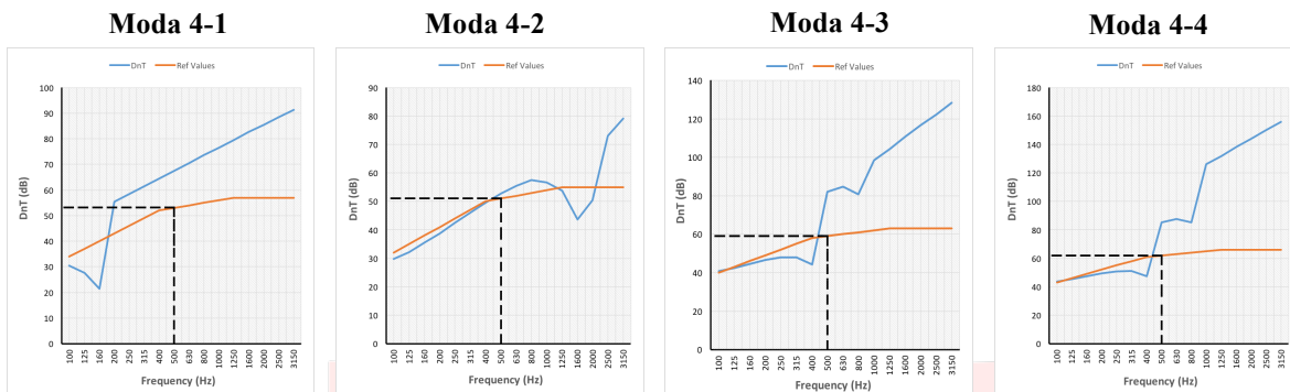
Gambar 9 Plot kurva D_{nT} dan kurva referensi tiap moda pada simulasi perancangan Dinding 4
