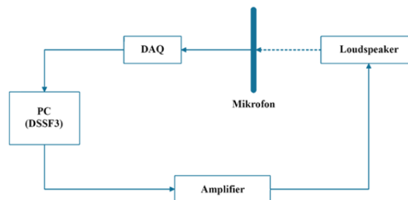
Gambar 3 Diagram blok konfigurasi alat ukur
