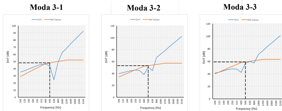
Gambar 8 Plot kurva D_{nT} dan kurva referensi tiap moda pada simulasi perancangan Dinding 3
