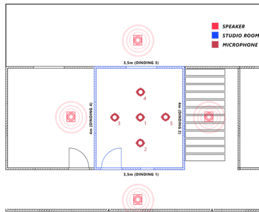
Gambar 4 Denah pemetaan 5 titik pengukuran
