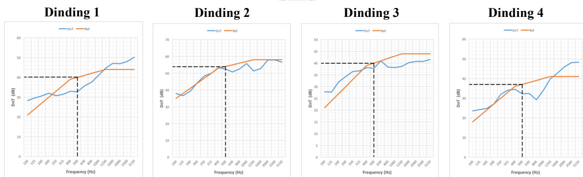
Gambar 5 Plot kurva D_{nT} dan kurva referensi pada setiap dinding ruangan
