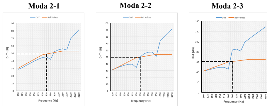
Gambar 7 Plot kurva D_{nT} dan kurva referensi tiap moda pada simulasi perancangan Dinding 2
