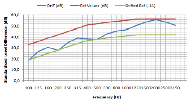
Gambar 1 Perbandingan kurva D_{nT} dengan kurva referensi.
