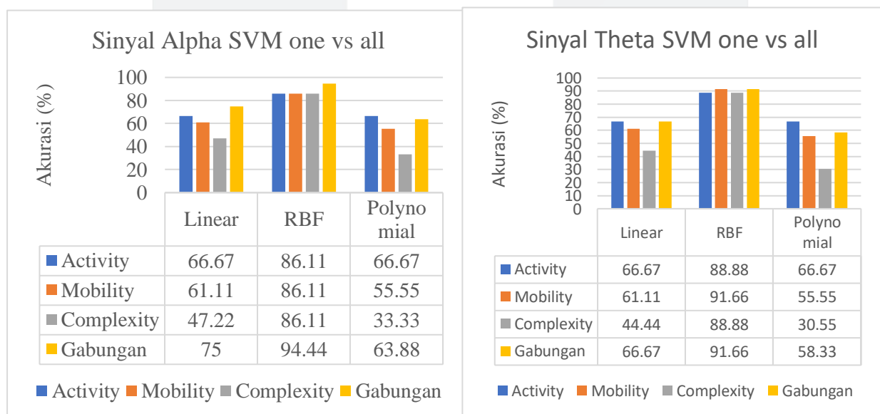
Gambar 4.6 Hasil pelatihan beberapa SVM metode one vs all
