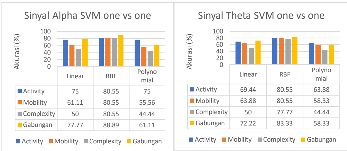
Gambar 6 Hasil pelatihan beberapa SVM metode one vs one
