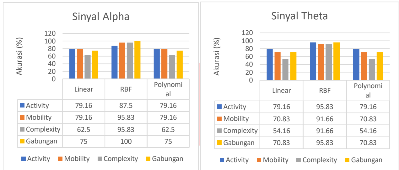
Gambar 5 Hasil pelatihan dengan beberapa SVM
