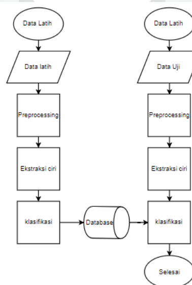
Gambar 2. Tahapan pelatihan dan pengujian sistem
