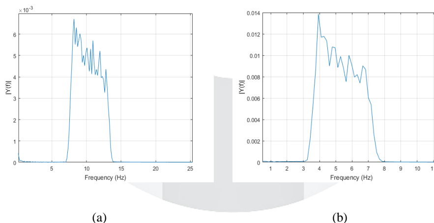
Gambar 4 Sinyal alpha (a) dan theta (b) pada domain frekuensi
