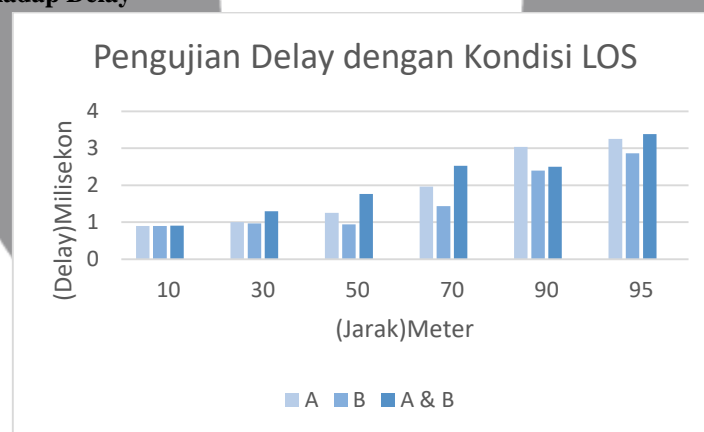
Gambar 5. Grafik Hasil Pengujian Delay
