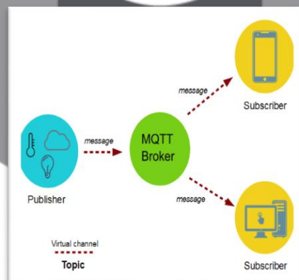
Gambar 2. Arsitektur MQTT
