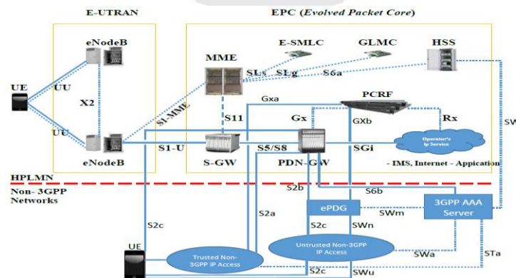
Gambar 2.2 Arsitektur LTE-A
