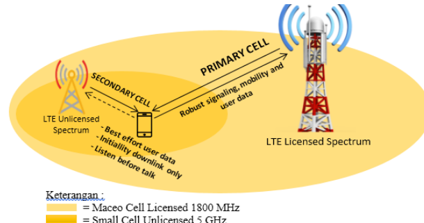
Gambar 2.3 Konsep LAA
