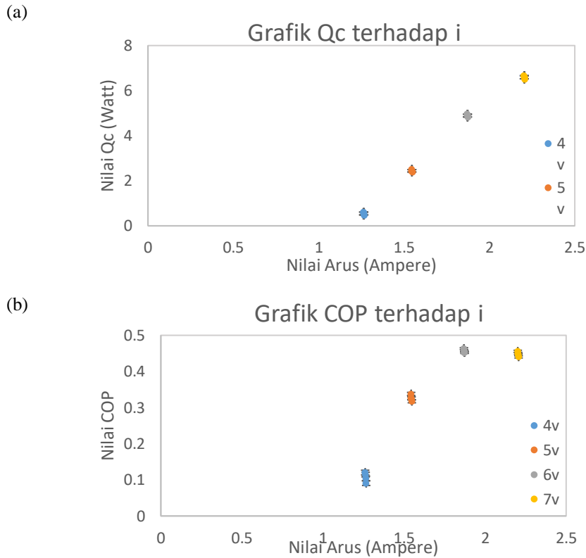
Gambar 3.4 (a) Grafik Q_c thd i , (b) Grafik COP thd i
