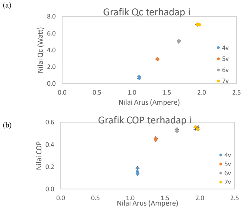
Gambar 3.1 (a) Grafik Q_c thd i , (b) Grafik COP thd i
