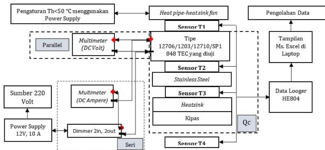
Gambar 2.2 Skema pengukuran alat uji
