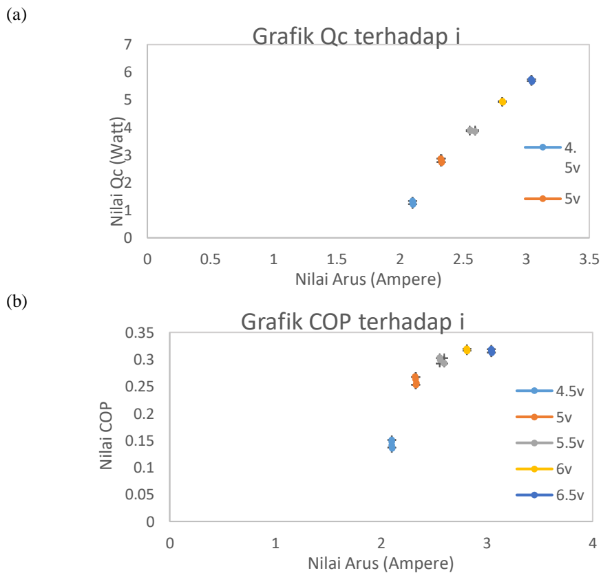
Gambar 3.3 (a) Grafik Qc thd I, (b) Grafik CP thd i
