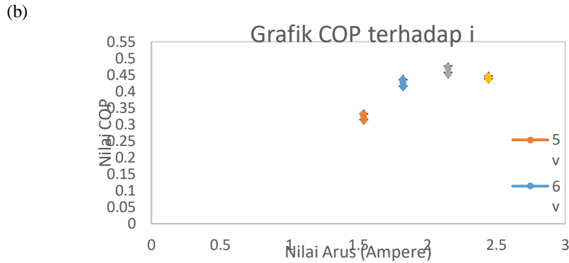
Gambar 3.2 (a) Grafik Qc terhadap i, (b) Grafik COP terhadap i
