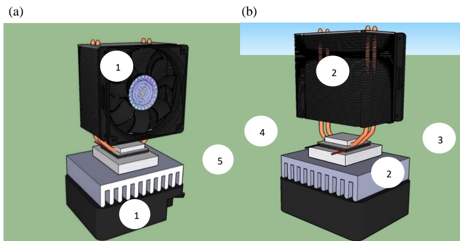
Gambar 2.1 Perancangan alat uji TEC. (a) Tampak depan, (b) Tampak belakang
