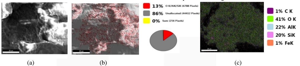
Gambar 3. Struktur permukaan dan komposisi unsur pada sampel tanah dengan resolusi 20 μm (a) Struktur umum (b) Struktur spesifik (c) komposisi unsur
