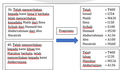
Gambar 3. Proses perubahan 2 hadits menjadi kode Soundex
